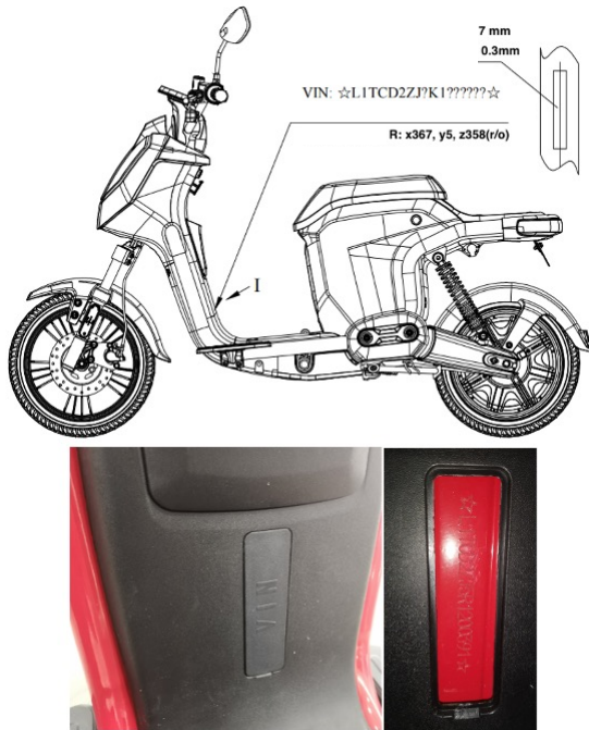
Fig. 4 VIN number
