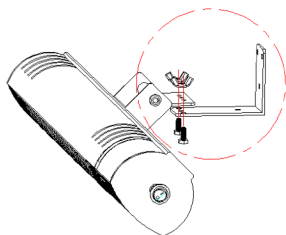
Schemat instalacji
